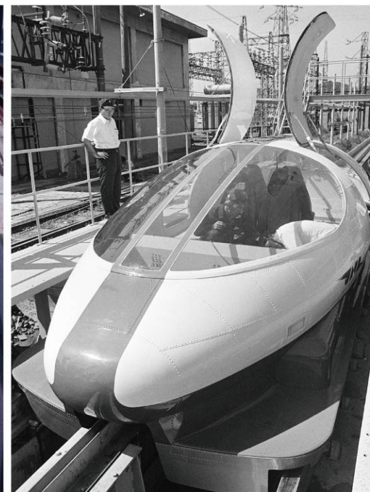
下左：リニアモーターカーの実験センター（宮崎）（撮影日：1978年07月05日） 下右：磁気浮上式列車公開実験。東京～大阪間を1時間で結ぶリニアモーターカーの実験車両。（東京・国分寺市光町の国鉄鉄道技術研究所）（撮影日：1972年09月19日） 写真：時事
